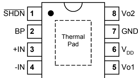
SOP8, MSOP8
